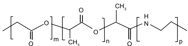
PLGA-PEI
