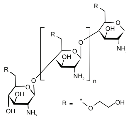
Glycol chitosan
