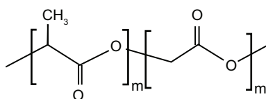
PLGA
