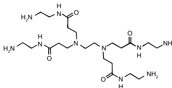
PAMAM dendrimer
