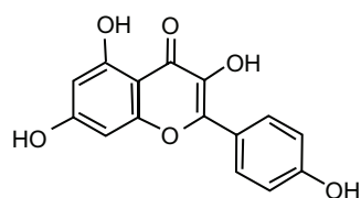
Kaempferol
